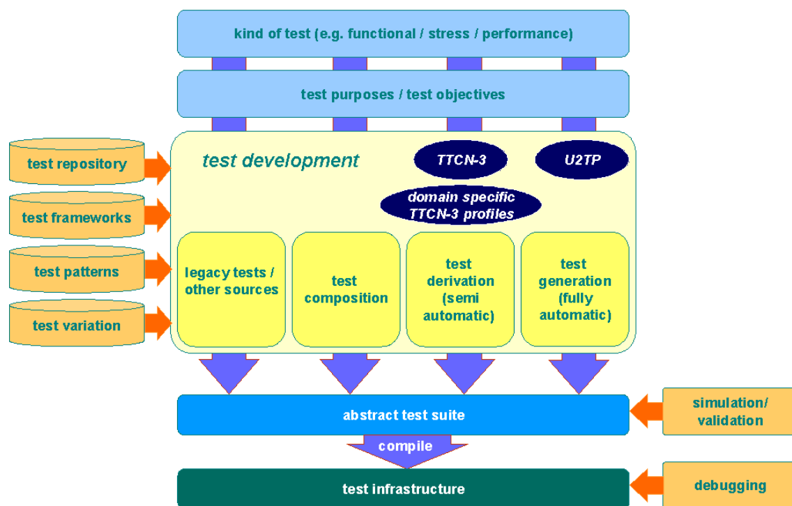
Abb. 5. Komponenten der Test-Plattform
