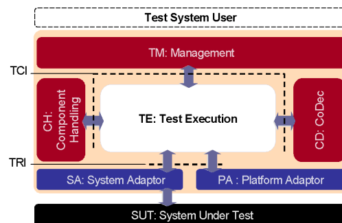
Abb. 2: TTCN-3 Ausführungsschnittstellen
