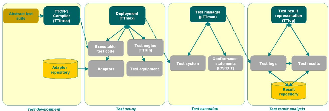
Abb. 4. Komponenten der Test Infrastruktur
