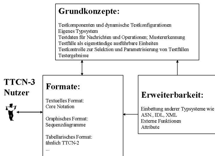
Abb. 1: TTCN-3 Überblick
