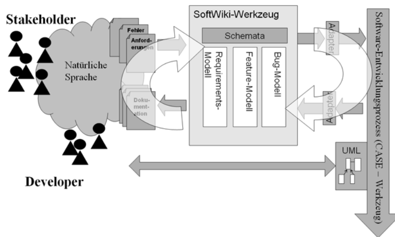
Abbildung 2: SoftWiki-Lösungsarchitektur
